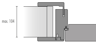
per muri sp. max. 104 mm
