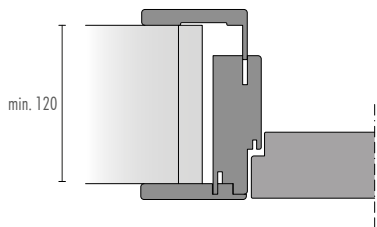
per muri sp. min. 120 mm
