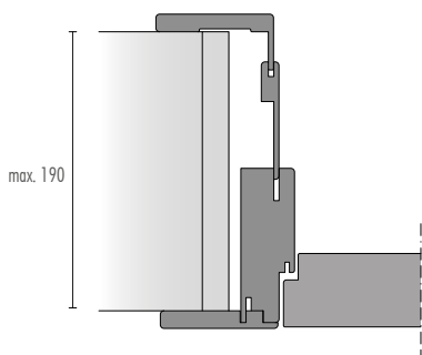
per muri sp. max. 190 mm
