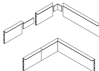
Соединительные элементы плинтуса MINI
