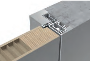
АЛЬДА-60 | ALDA-60, короб ИНВИЗИБЛ | INVISIBLE
