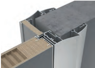
короб ДЭКО | DECO
