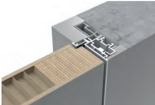
ЛЭВЭЛ-60 | LEVEL-60, короб ИНВИЗИБЛ | INVISIBLE
