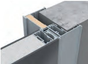
короб ПЛАНАР | PLANAR
