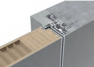
короб ИНВИЗИБЛ | INVISIBLE
