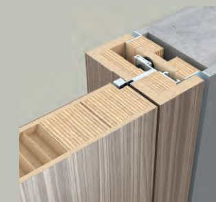
Полотно, наличник, короб и стена в одной плоскости
