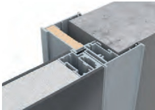
короб ПЛАНАР | PLANAR
