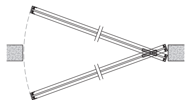
PIVOT-СЛИМ, Трэ, GT02 Прозрачное Серое , AL08 Чёрный PIVOT-SLIM, Tre, GT02 Trasparente Grafite , AL08 Black
