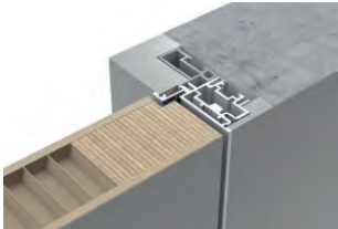
ТРЭНД-60 | TREND-60, короб ИНВИЗИБЛ | INVISIBLE
