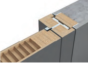
короб ЮНИВУД | UNIWOOD
