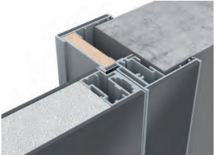
короб ПЛАНАР | PLANAR со вставкой
