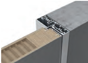
короб МАКСИ | MAXI
