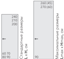
ЛЭВЭЛ-60 | LEVEL-60, короб МАКСИ | MAXI
