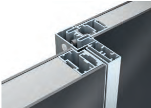
ВОЛСТРИТ-ЛАГО | WALLSTREET-LAGO с дверным коробом
