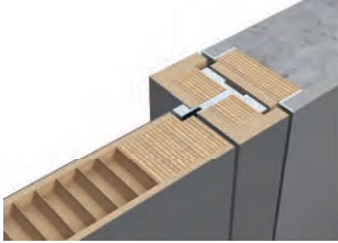
короб ЮНИВУД | UNIWOOD
