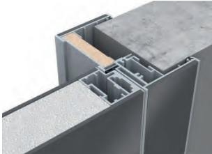
короб ПЛАНАР | PLANAR со вставкой
