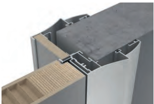
ТРЭНД-60 | TREND-60, короб ДЭКО | DECO
