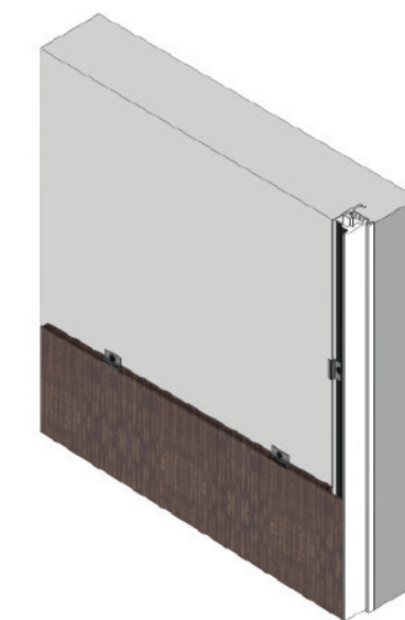
Ancoraggio pannello iniziale Boiserie-H.
