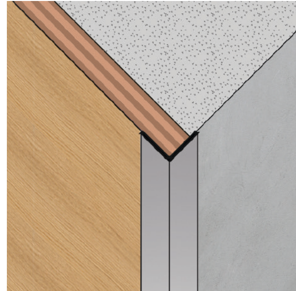
Profilo in alluminio laccato o in tinta per chiusura terminale.
