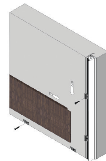
Installazione pannello iniziale Boiserie-H.
