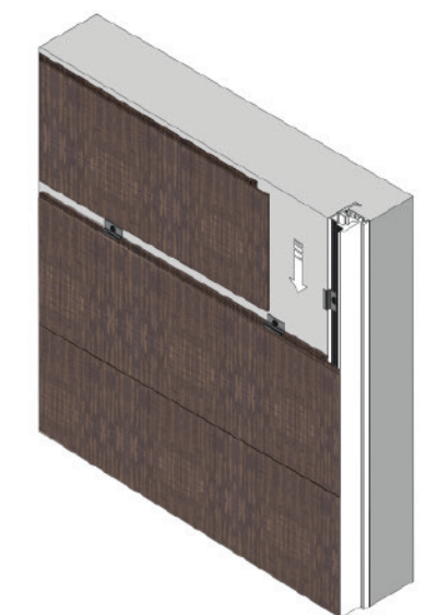
Installazione pannelli successivi Boiserie-H.
