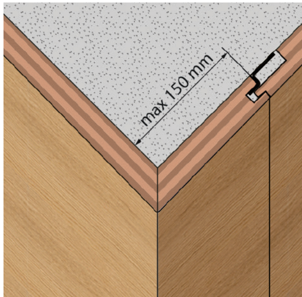
Pannello assemblato a 45° con un lato di dimensione max 150 mm.
