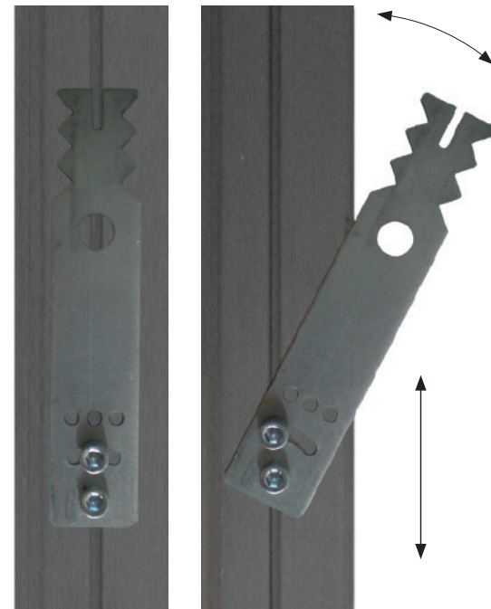
Zanca regolabile in altezza e profondità. The waltie is adjustable in height and depth.
