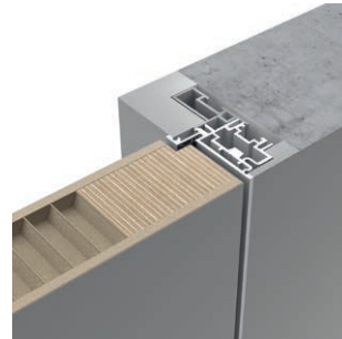
TREND-60, короб INVISIBLE
