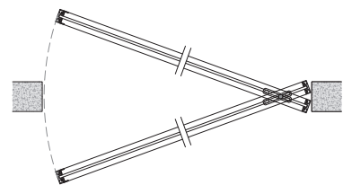
PIVOT-45. Фиксация в положении "закрыто" и положении "открыто" с двух сторон.
